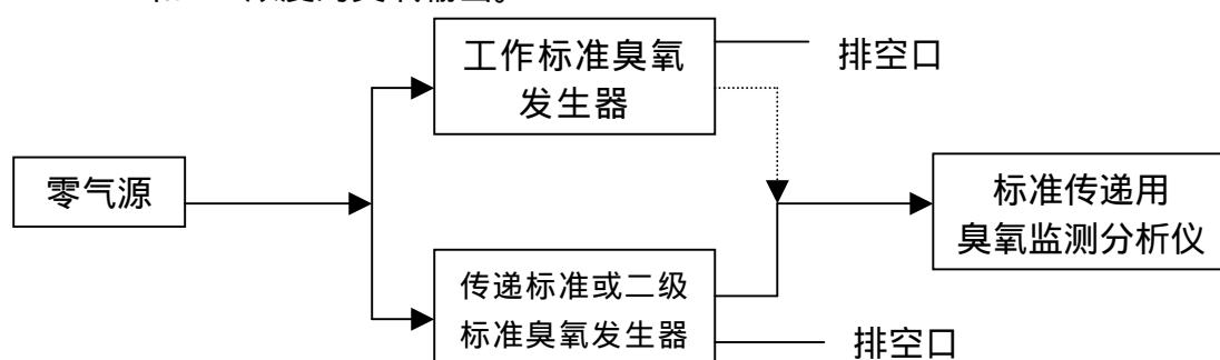
图 C1.4 臭氧发生器标准传递图
