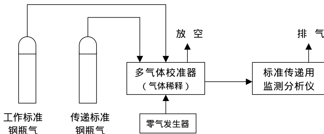
图 C2.2 钢瓶标准气传递法图
