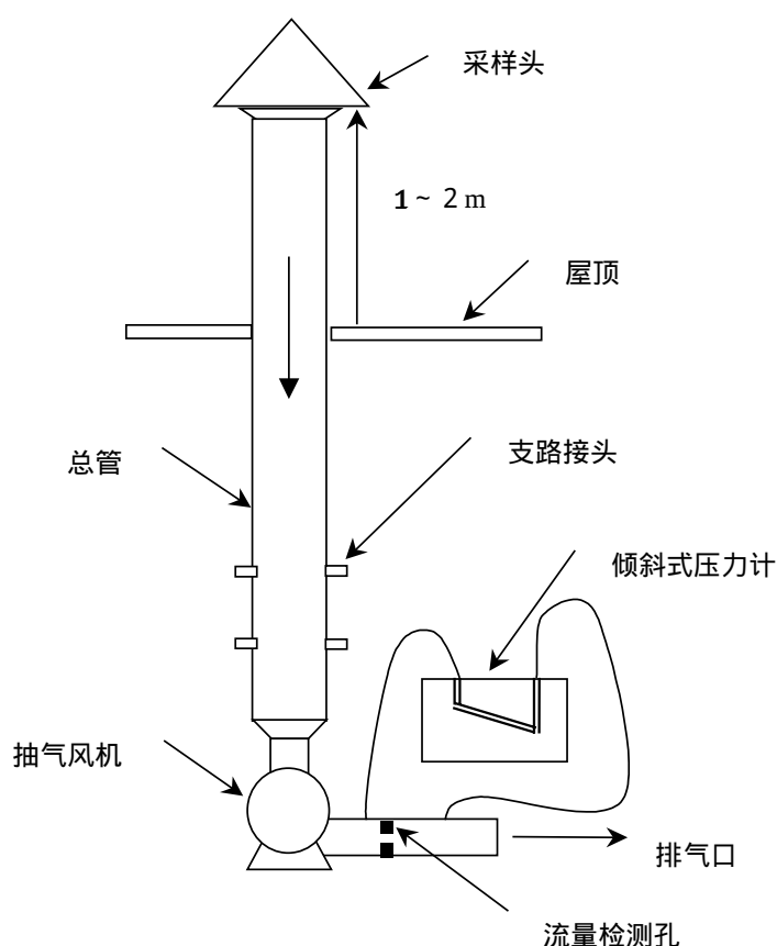
图 4.2.1 垂直层流多路支管系统
