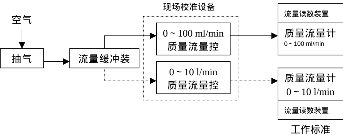
图 C1.2 质量流量控制器标定图
