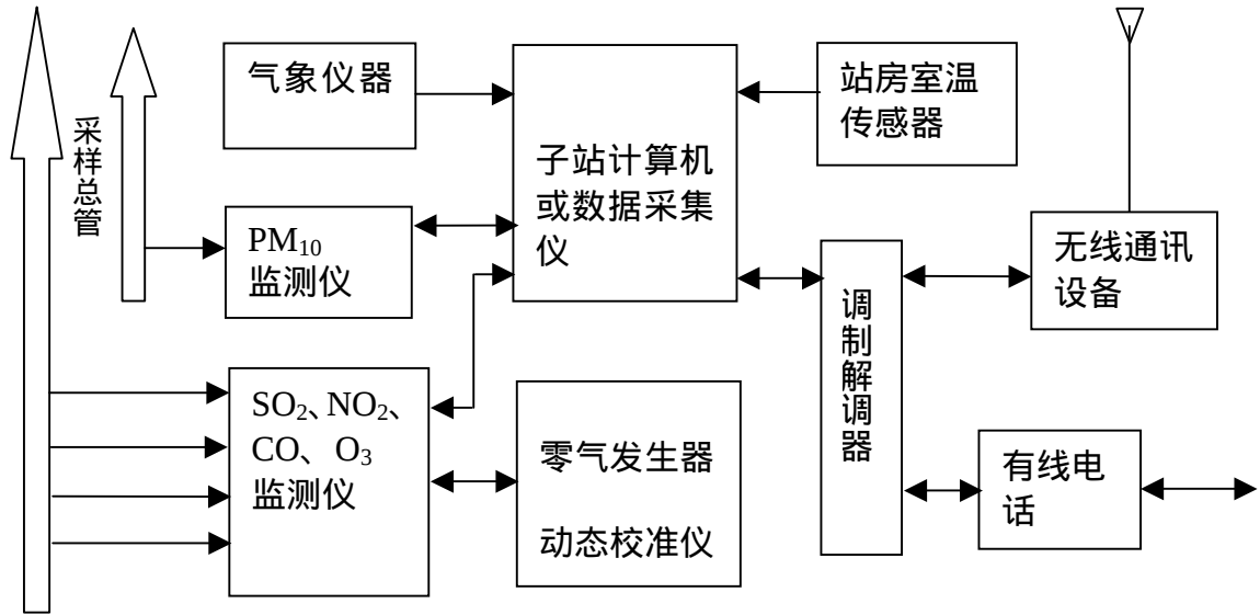
图 4.7.1 监测子站仪器设备配置示意图
