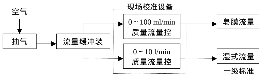
图 C1.3 流量传递与校正系统图
