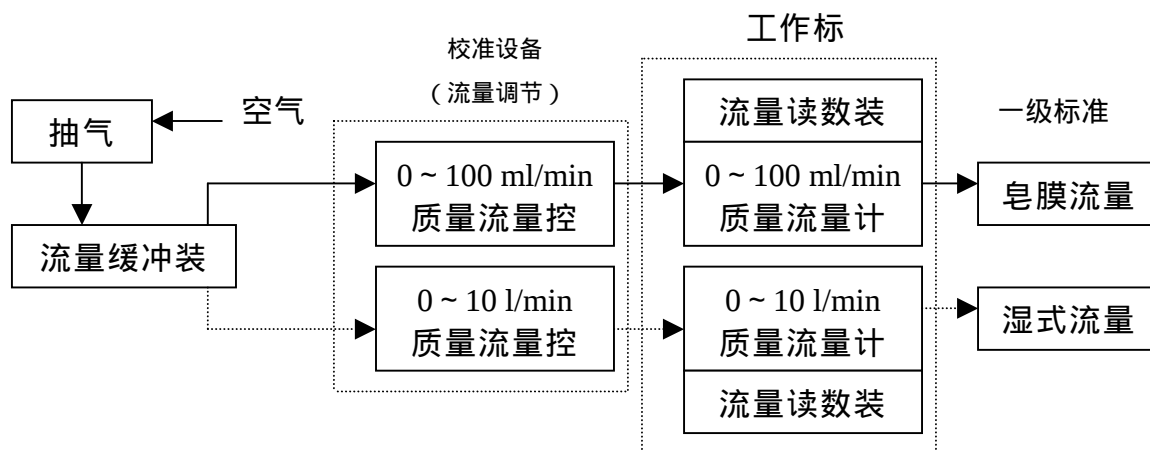
图 C1.1 流量传递和校正仪器连接图
