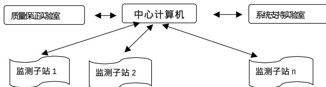
图 4.1.1 环境空气质量自动监测系统基本构成框图
