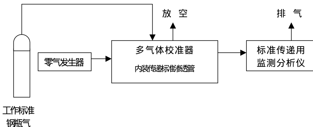
图 C2.3 渗透管传递图
