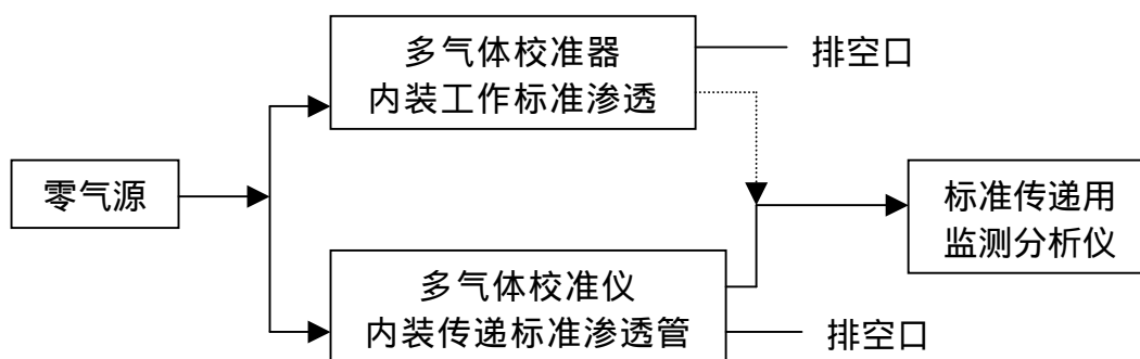
图 C2.1 传递仪器校准图
