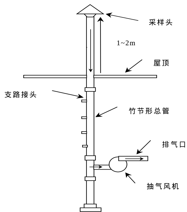
图 4.2.3 竹节式多路支管系统(2)
